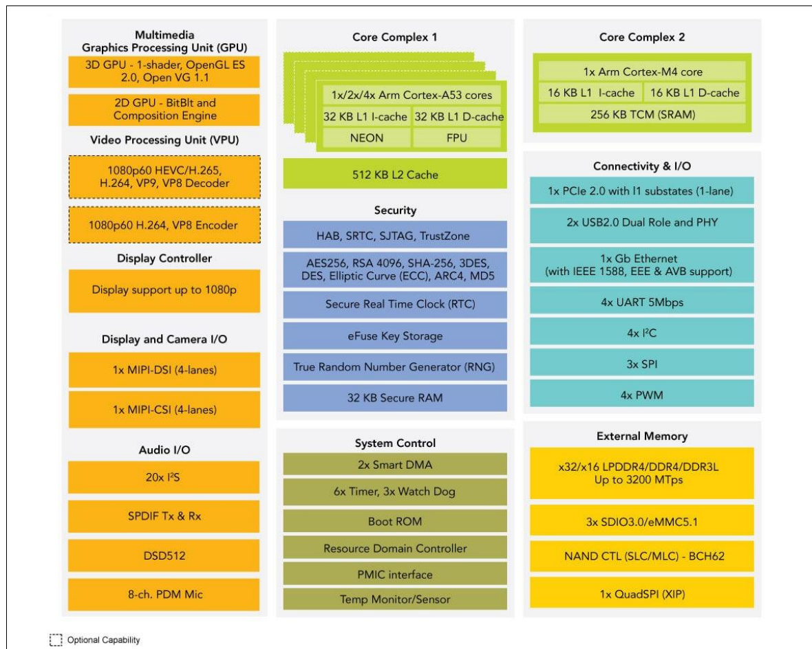
Figure 2 i.MX8M Mini Block Diagram
